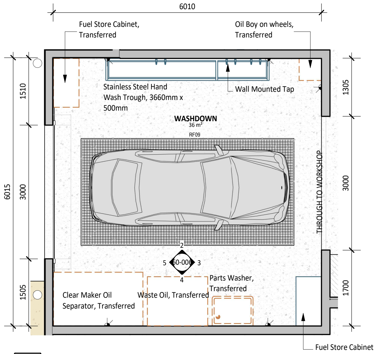
1 PLAN DETAIL 30-01 1 : 50
